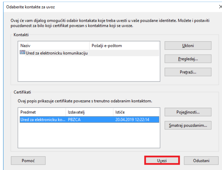
Slika 8 - Uvoz certifikata
