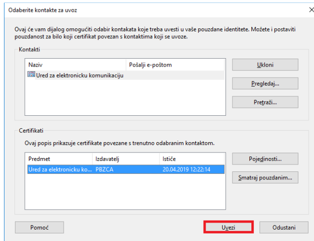
Slika 6 - Odabir certifikata
